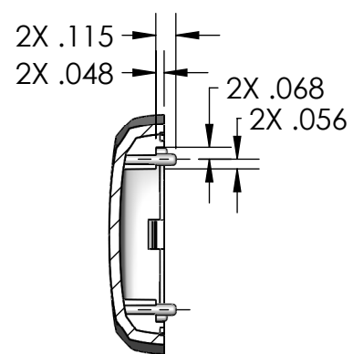
SECTION D-D
