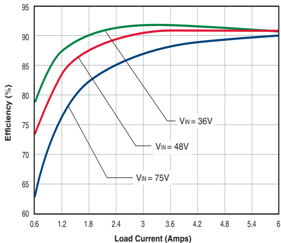
UVQ-18/6-D48N
