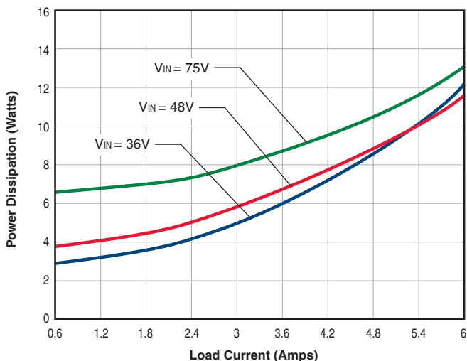
UVQ-18/6-D48
