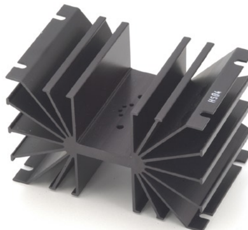
HS04 0.95°C/W
