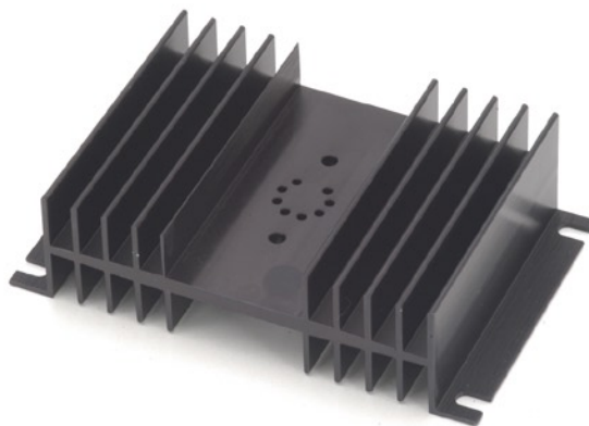
HS03 1.7°C/W
