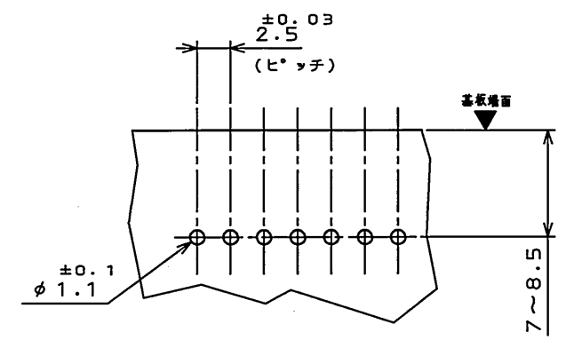
△ 基板取付穴寸法(参考)
