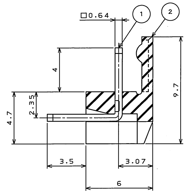
断面 A-A
